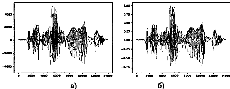
Рис.5. Оцифрованный речевой сигнал до (а) и после (б) нормализации
