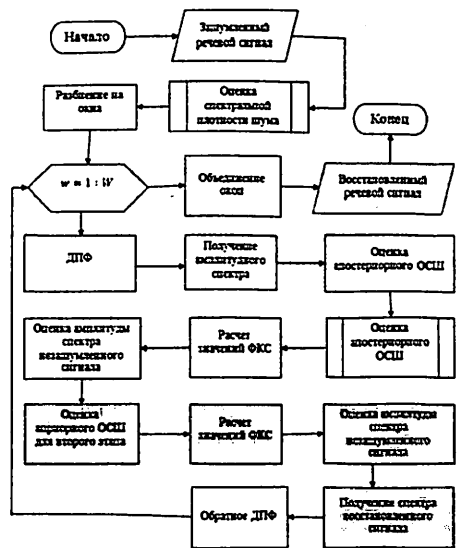
Рис.7. Блок-схема двухэтапного алгоритма шумоподавления
