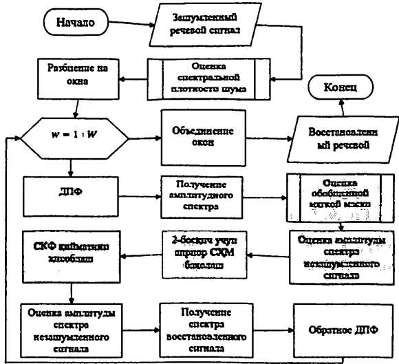
Рис.8. Блок-схема алгоритма шумоподавления на основе мягких масок
