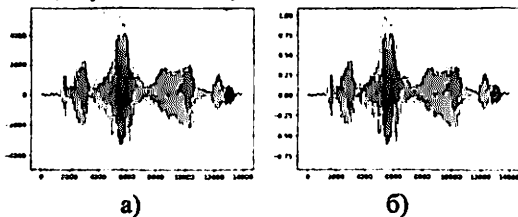
5-расм. Нормаллаштиришгача (а) ва нормаллаштиришдан сўнг (б) рақамлаштирилган нутқ сигнали
