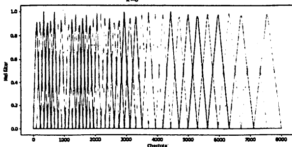
Рис.3. АЧХ мел-фильтров Q=24
