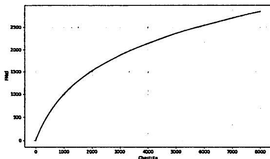
Рис.2. Соотношение частот обычной шкалы к частотам мел-шкалы
