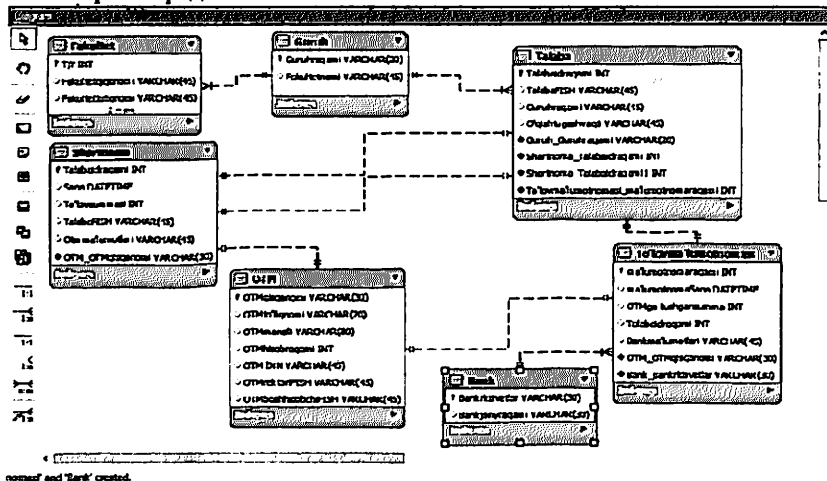
5-расм. Маълумотлар базасининг боғланишлар ва муносабатлар схемаси
