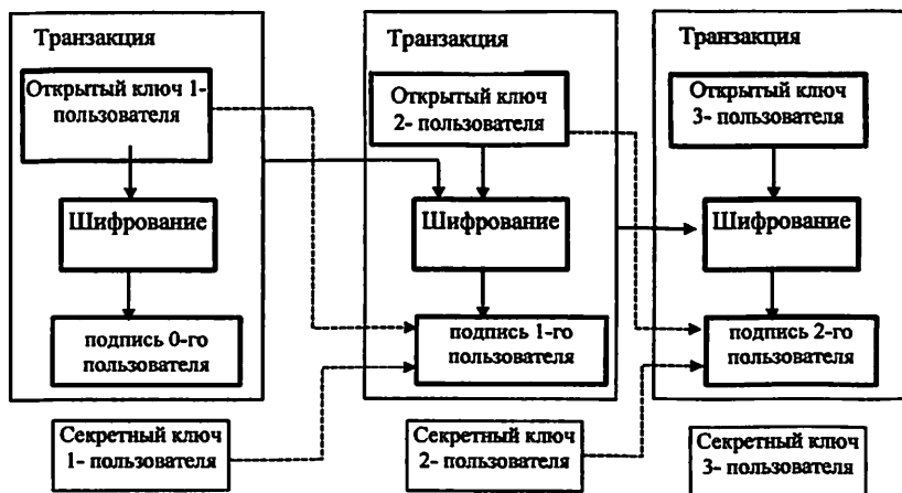
Рис. 1. Схема подтверждения правильного выполнения транзакции
