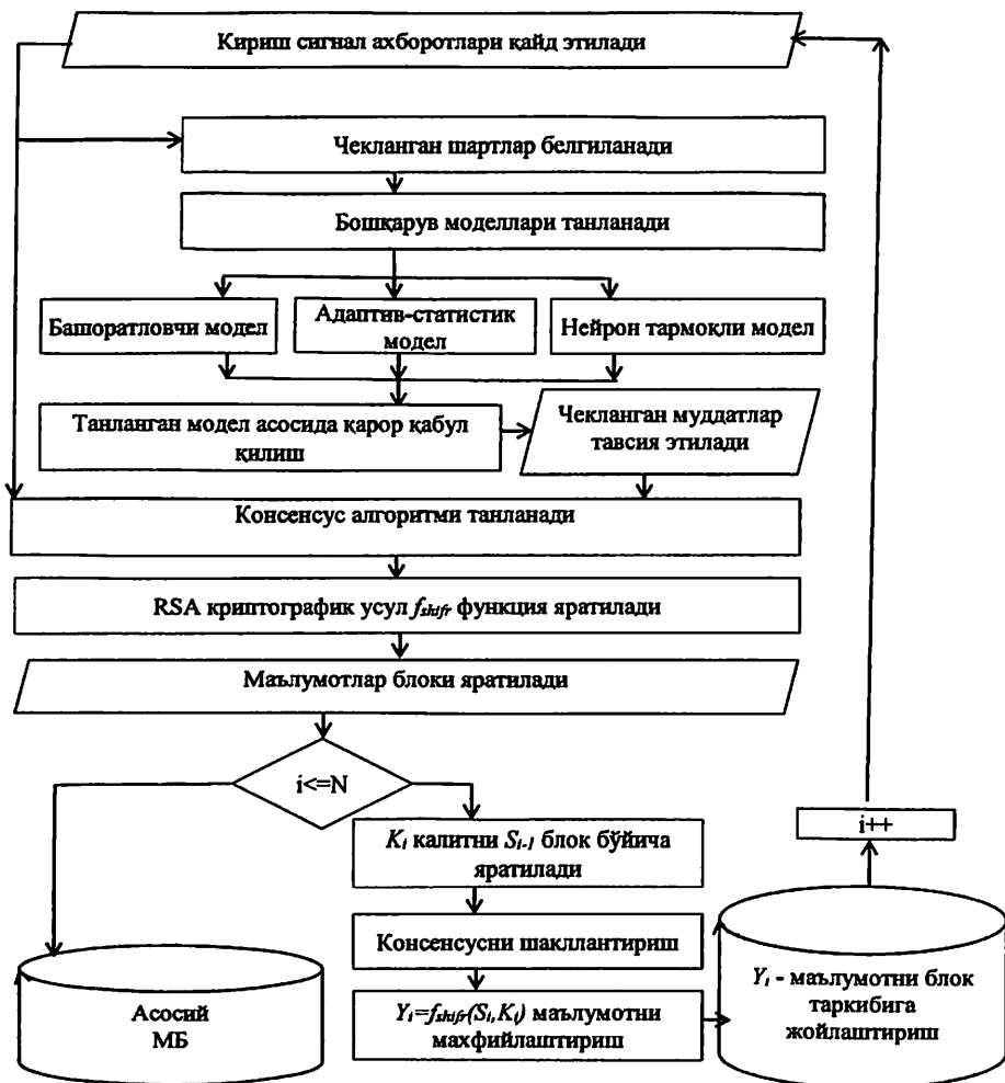
3-расм. Бошқарувни оптималлаштириш ва маълумотлар ишончлилигини ошириш дастурий мажмуасинининг умумий схемаси
