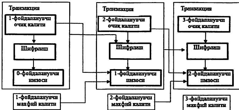
1- расм. Транзакция тўғри бажарилганлигини тасдиқлаш схемаси
