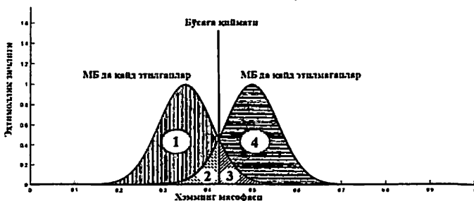
4-расм. Хэмминг масофасини қийматларининг шартли эҳтимоллик тақсимоли
