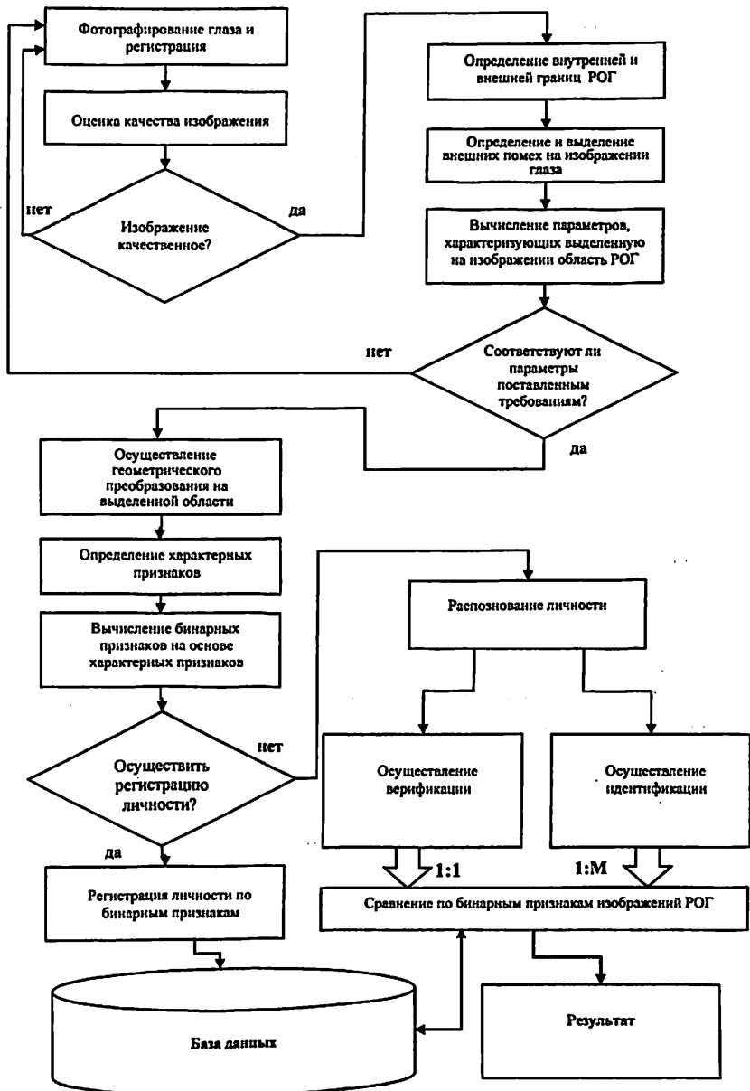
Рис. 5. Общая схема работы программного комплекса биометрической идентификации личности на основе анализе изображение радужной оболочки глаза (РОГ)
