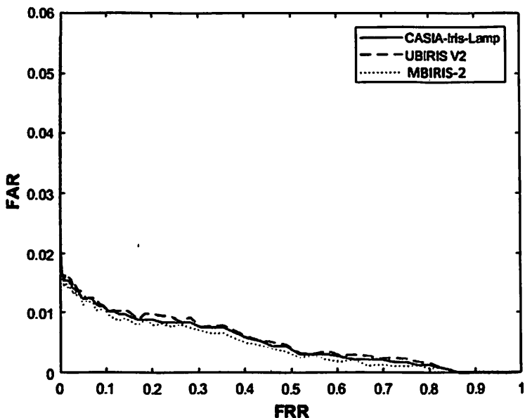
6-расм. 1-тур (FRR) ва 2-тур (FAR) хатоликлар боғлиқлигининг эгри чизиқлари
