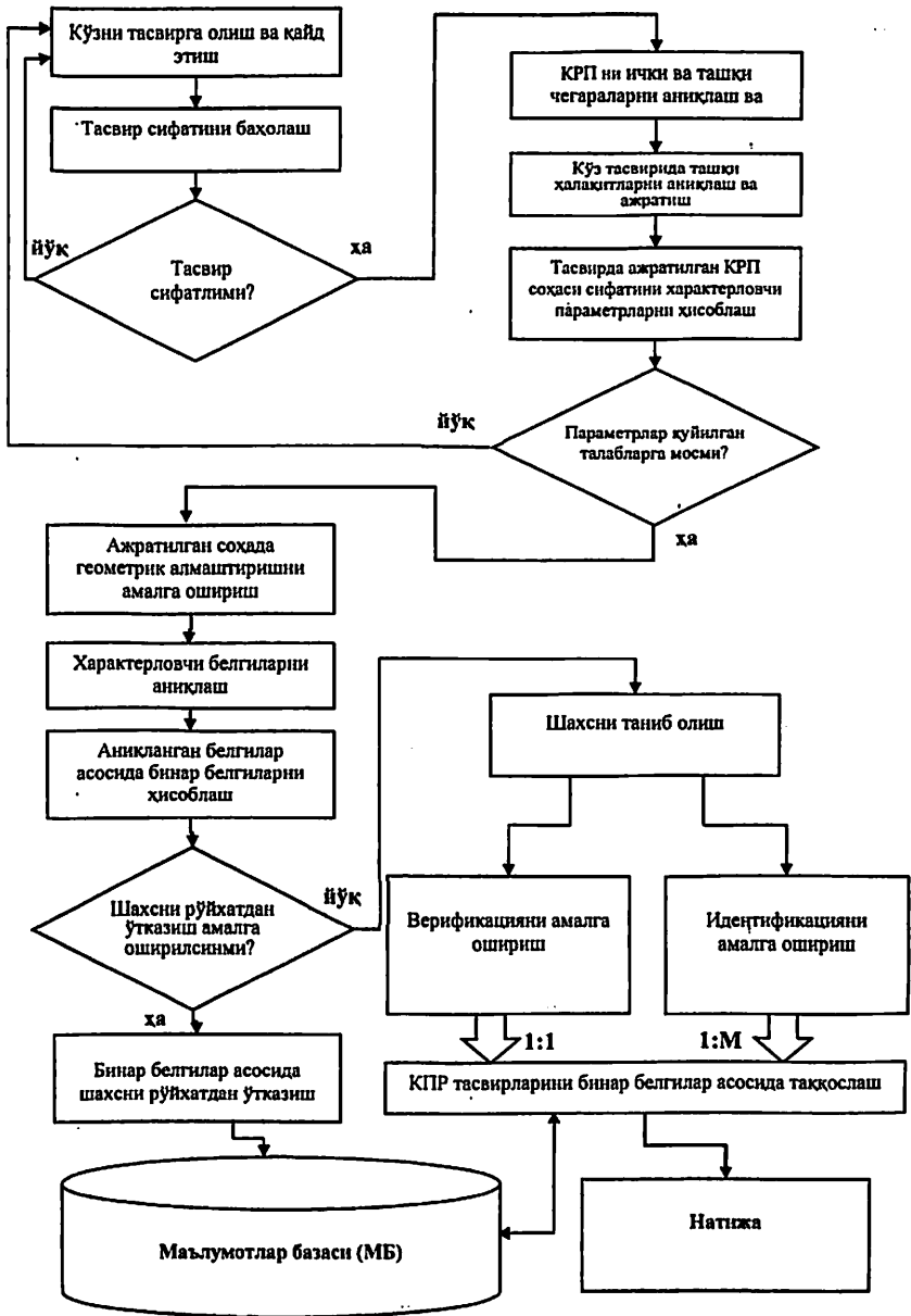
5-расм. Кузнинг рангдор пардаси (КРП) тасвири асосида шахсни биометрик идентификациялаш дастурий муҳрамини аниқловчи алгоритмнинг схемаси
