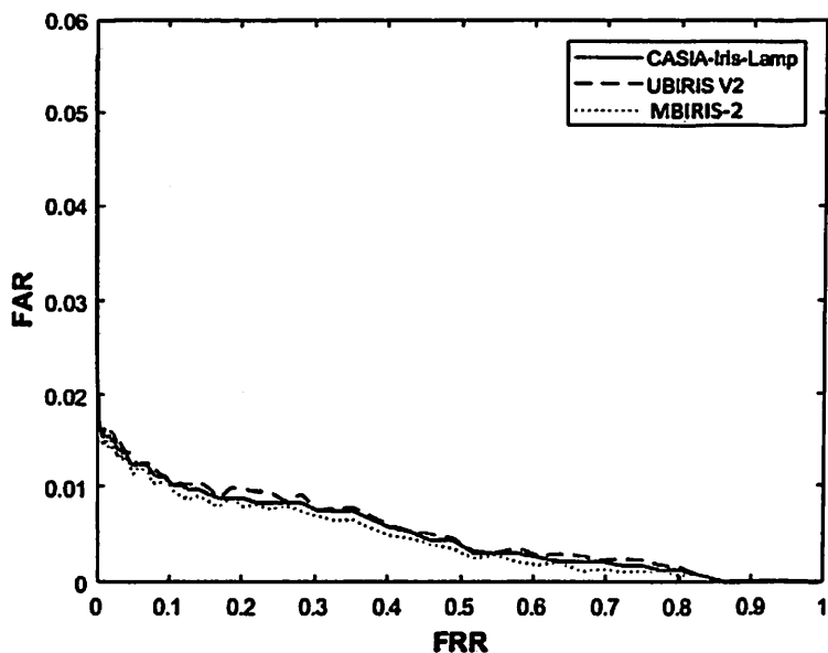
Рис. 6. Кривые зависимости ошибок первого рода (FRR) и второго рода (FAR)
