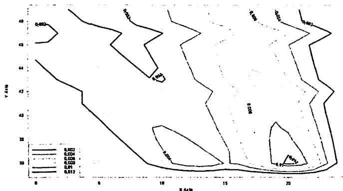
2-расм. Атмосферада зарарли моддаларнинг кўчиши ва диффузияси жараёнини тадқиқ қилиш учун қаралаётган ҳудуд орографиясини инobatга олган ҳолда ҳисоблаш тажрибалари натижаси ( z=10\text{ м} )
