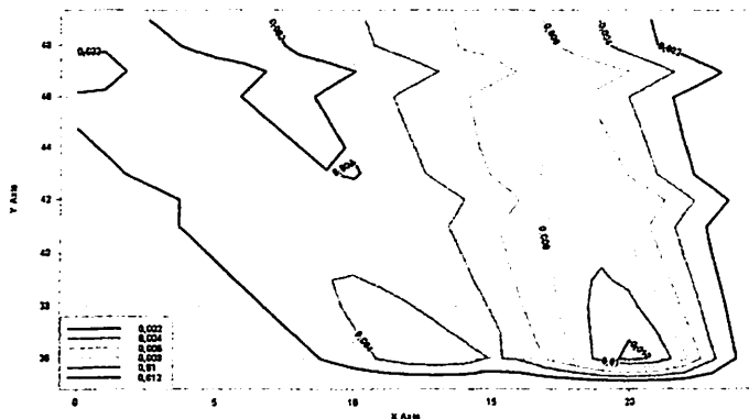
Рис. 2. Результаты вычислительных экспериментов по исследованию процесса переноса и диффузии вредных веществ в атмосфере с учетом орографии рассматриваемой местности ( z=10 м)
