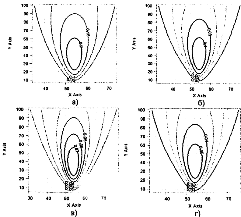
3 – расм. Олтингургурт оксиди (IV) зарарли моддасининг атмосферада кўчиши ва диффузияси жараёнини шамолнинг турли тезликларида визуализация қилиш ( PЭМК=0,05\text{ мг/м}^3 ).
