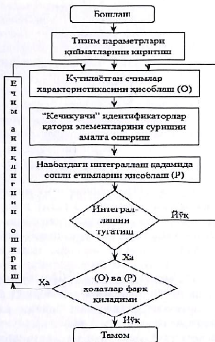
3-расм. (10) тенгламани ШҚда амалга ошириш блок-схемаси
