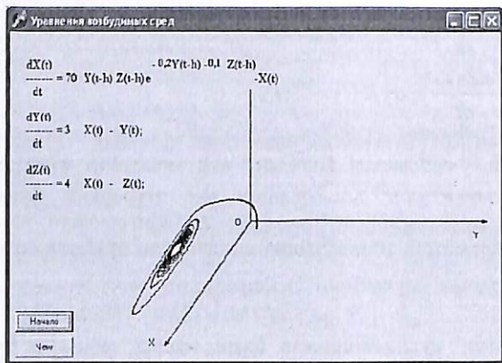
1-расм. Кўзгалувчан мухит минимал базис модел тизимининг Пуанкаре типдаги лимит цикли
