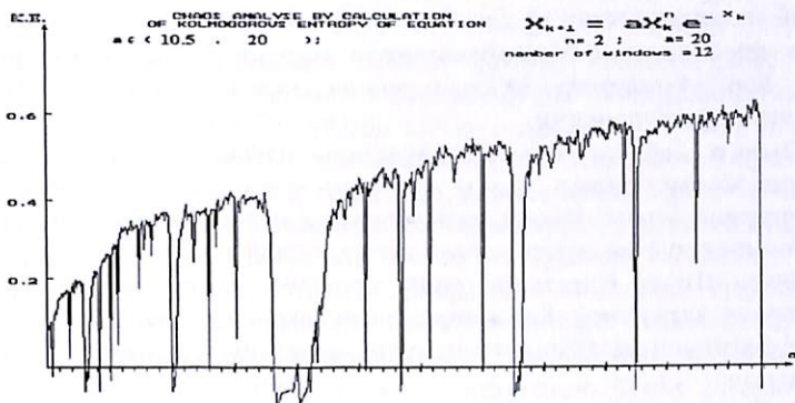
2-расм. (14) да динамик хаос соҳаси рельефи
