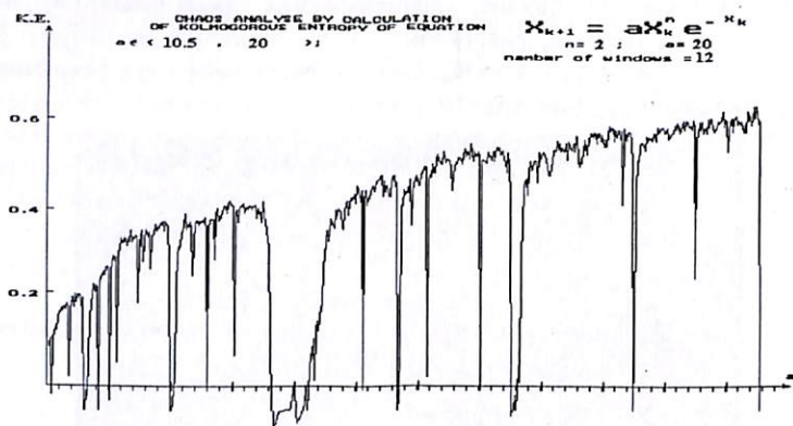
Рис. 2. Рельеф области динамического хаоса в (14)
