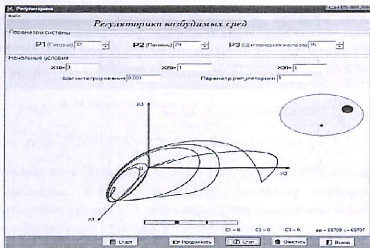
4-расм. «Юрак-жигар-қалқонсимон без» тизимида «қора ўрама» ҳолати
