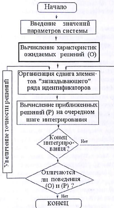
Рис. 3. Блок-схема реализации уравнений (10) на РС
