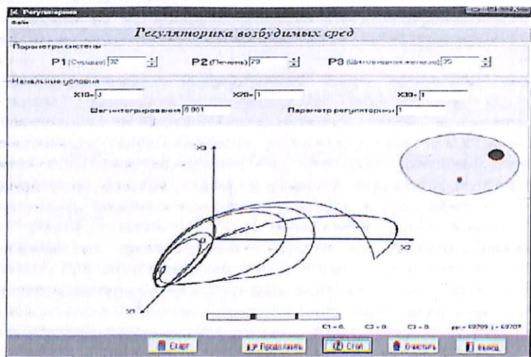
Рис. 4. Эффект «черная дыра» в компьютерной модели биосистемы «сердце-печень-щитовидная железа»
