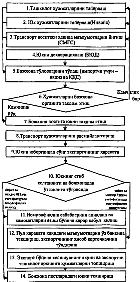
2 расм. Темир йўл импорт ва экспорт юкларининг божхона жараёнларини амалга ошириш алгоритми
