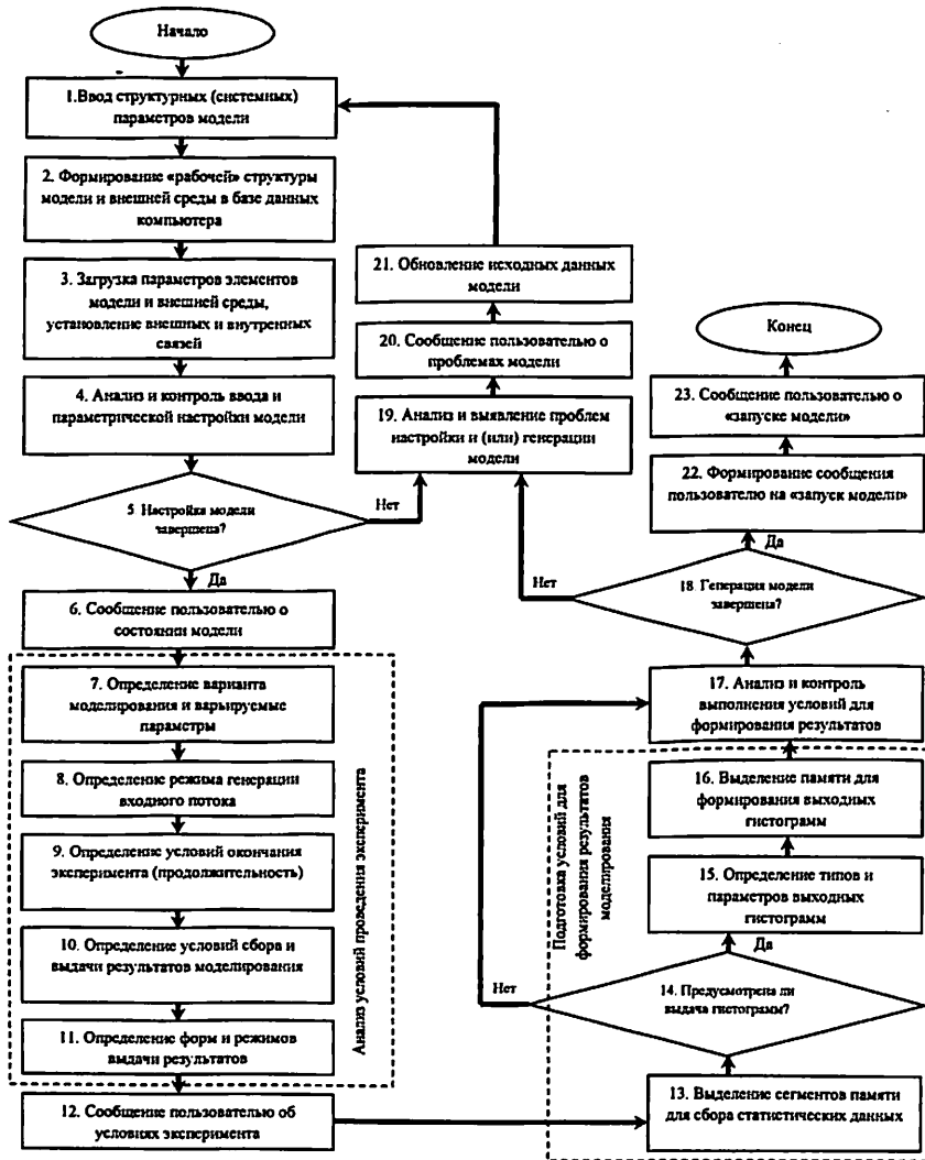
Рисунок 3. Алгоритм этапов создания модели таможенного контроля
