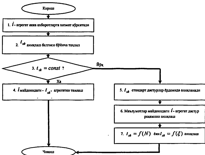
5 расм. Агрегат хабарларини хизмат кўрсатиш вақтини аниқлаш алгоритми
