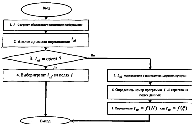
Рисунок 5. Алгоритм определение времени оказания услуг агрегат информации.
