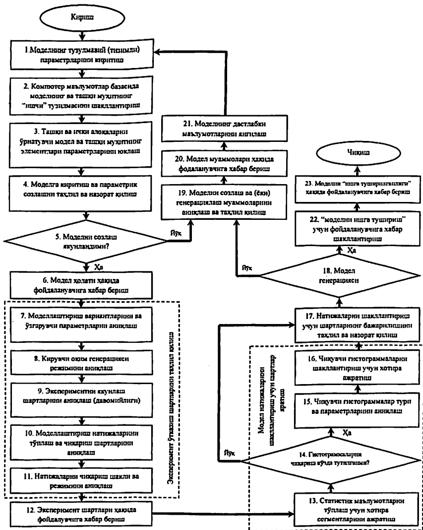
3 расм. Божхона назорати моделини яратиш босқичлари алгоритми
