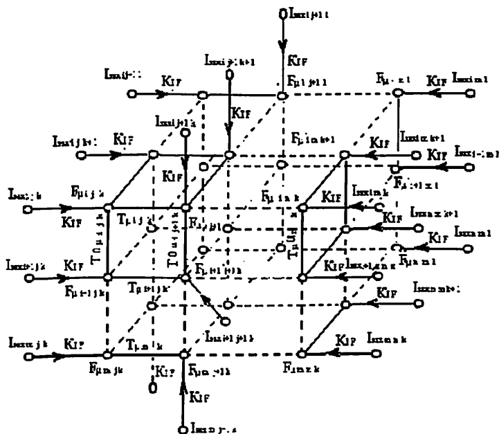
Рис.2. Графовая модель магнитной системы преобразования электромагнитных преобразователей тока в напряжение с плоскими измерительными обмотками
