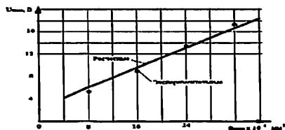
Рис.9. Зависимость выходного напряжения U_{\text{вых}} от различных значений площади сечения S_{\text{плн}}
