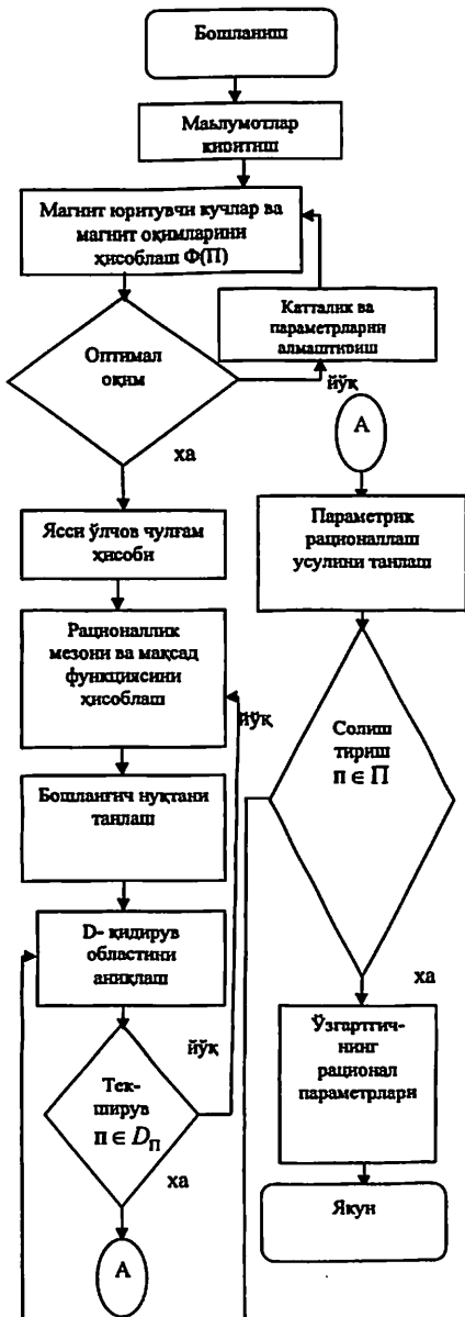
14-расм. Рационал параметрларини аниқлаш алгоритми блок-чизмаси
