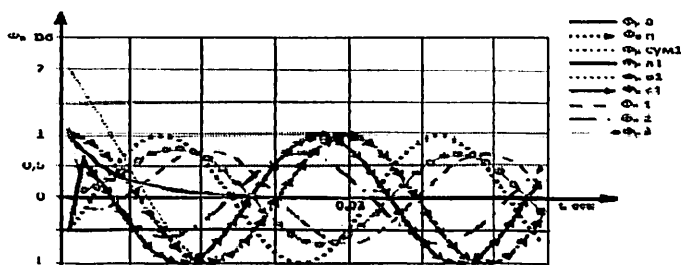
10 - расм. Энерготизим уч фазали электр тармоғида тоқлар оқими ҳосил қилган ясси ўлчов чулғамли токни кучланишга электромагнит ўзгартириш магнит тизимидаги оқимларнинг қийматлари
