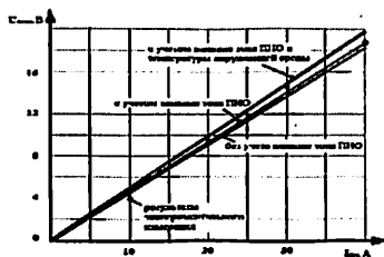
Рис.12. Влияние I_{вых} и T_m на выходное напряжение U_{вых}
