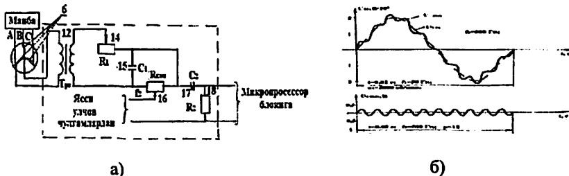
18-расм. Реактив қувват динамик манбасини айланиш тезлигини назорат қилиш ва бошқариш чизмаси (а) ҳамда ясси ўлчов чулғамли токни кучланишга электромагнит ўзгартгичларнинг чиқиш таснифлари (б)
