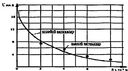
7 - расм. U_{\text{эчик}} чиқиш кучланишининг \delta нинг қийматларига боғлиқлиги
