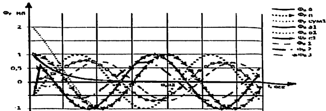
Рис.10. Изменение магнитных потоков в магнитной системе электромагнитных преобразователей тока в напряжении с плоскими измерительными обмотками при протекании токов по трехфазной электрической сети энергосистем
