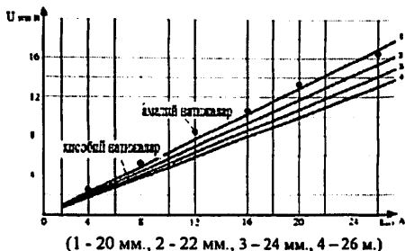
6- расм. \delta ҳаво оралиқнинг қийматларида статик таснифлар
