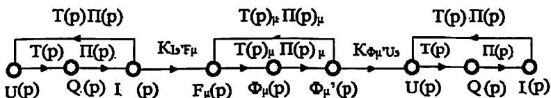
Рис. 3. Динамическая графовая модель электромагнитных преобразователей тока в напряжение с плоскими измерительными обмотками
