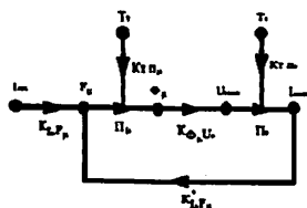
11 - расм. Ҳатолик манбаларини тадқиқоти граф модели
