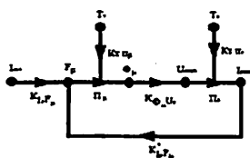
Рис.11. Графовая модель для исследования источников погрешностей
