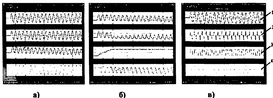
Рис.5. Изменения входного (1 – первичный ток - I_{нр} ), промежуточных (2 – м.д.с. F_p и 3- магнитного потока - \Phi_p ) и выходного (4 – вторичное напряжение U_{нр} ) величин электромагнитных преобразователей тока в напряжение с плоскими измерительными обмотками при: нормальном (а), несимметричном (б) режимах и в режиме короткого замыкания (в)
