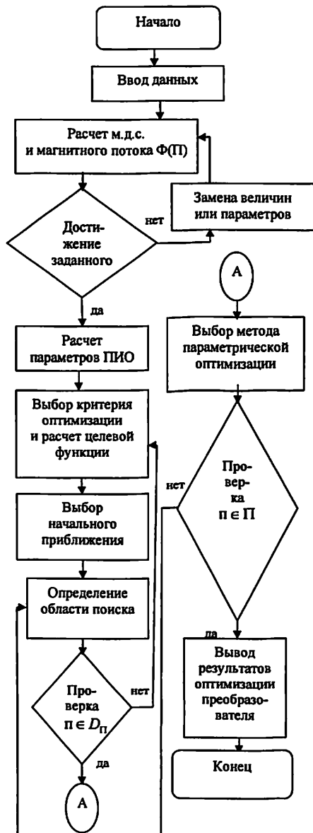
Рис.14. Блок-схема алгоритма оптимизации параметров
