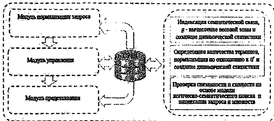
Рис. 2. Общая функциональная структура СИС в поисково-информационной системе.
