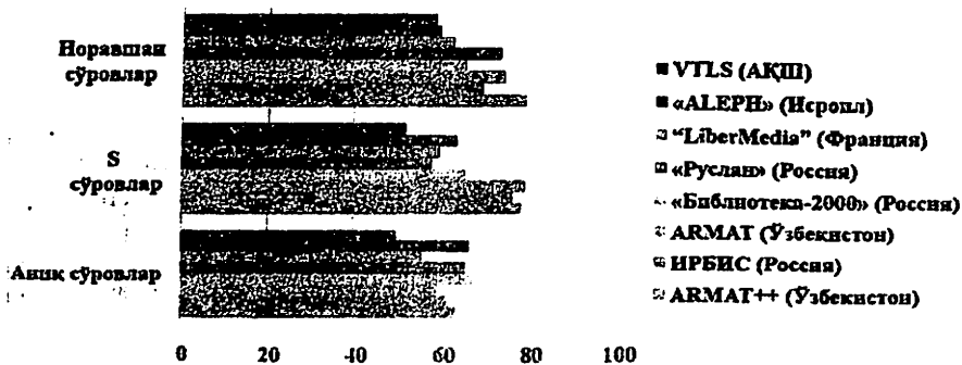
6-расм. Маълумотларни излаш ва қайта ишлашнинг «Тезлик» параметри бўйича натижалари.
