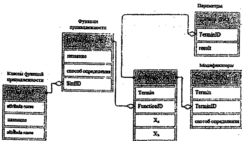
Рис. 3. IDEF1x модель ядра базы знаний.
