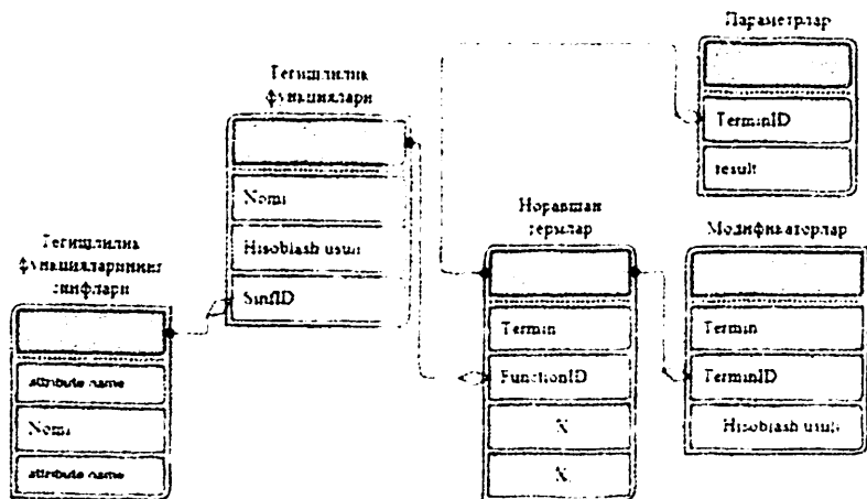
3-расм. Билимлар базасининг ядросини IDEF1x модели.
