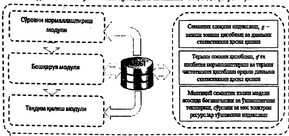
2-расм. САМда маълумотларни излаш тизимининг умумий функционал тузилмаси.
