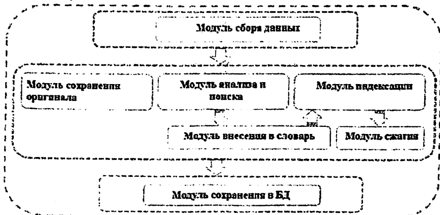
Рис. 2. Функциональная структура программного модуля сохранения данных.
