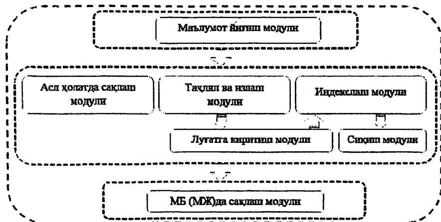
2-расм. Маълумотларни сақлаш дастурий модулининг функционал тузилмаси.
