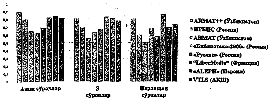
7-расм. Маълумотларни излаш ва қайта ишлашнинг «Долзарбликнинг ўрта қиймати» параметри бўйича натижалари.
