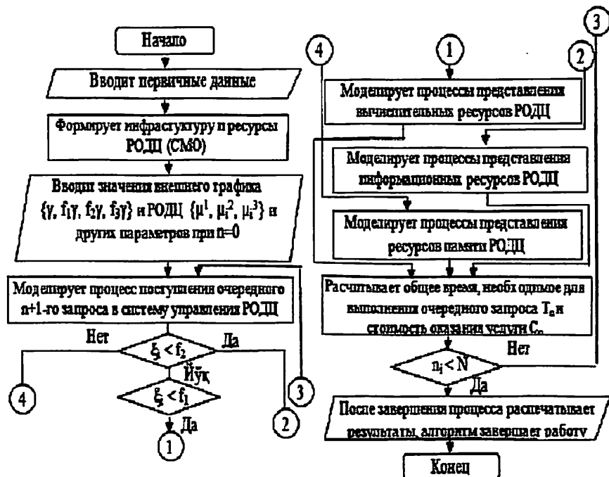
Рис. 3. Алгоритм моделирования процессов формирования и представления ресурсов РОДЦ
