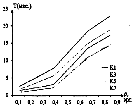
Рис. 5. Диаграмма представления вычислительных ресурсов РОДЦ T=F(\rho)
