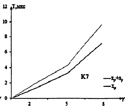
Рис. 7. Диаграмма вычисления и представления вычислительных и информационных ресурсов РОДЦ T=F(x_p, a_p)
