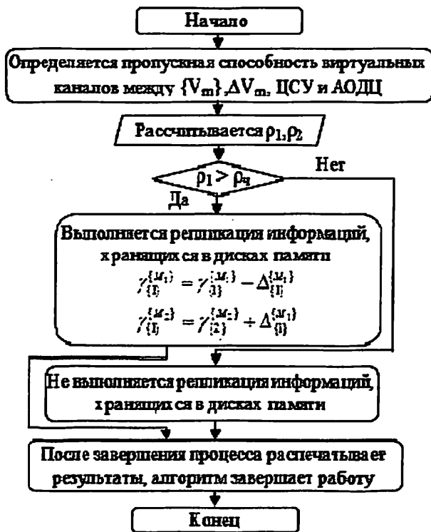
Рис. 2. Алгоритм размещения в хранилищах памяти РОДЦ на основе метода репликации
