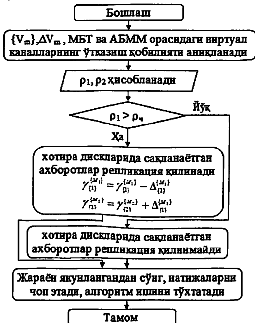
2-расм. ТБММ хотира омборларига репликация усули негизда жойлаштириш алгоритми
