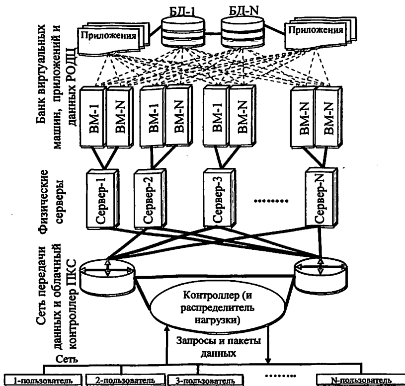
Рис.1. Концептуальная модель РОДЦ на основе ПКС
