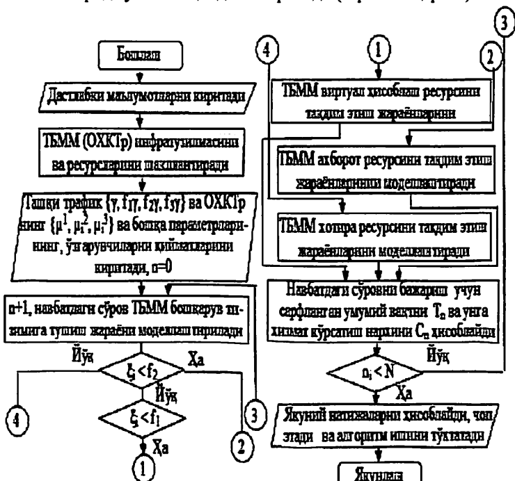
3-расм. ТБММ ресурсларини шакллантириш ва тарқатиш усулининг моделлаштириш алгоритми
