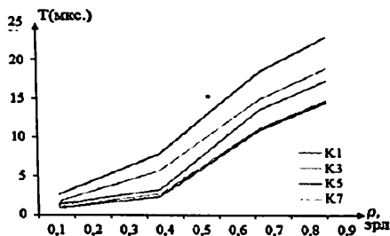
5-расм.ТБММ ҳисоблаш ресурсларини тақдим этиш T=F(\rho) диаграммаси
