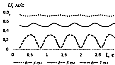
2-расм. Турли қатламларда зарра ҳаракати тезлигининг вақт бўйича ўзгариши.
