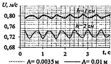
1-расм. Зарра ҳаракати тезликларининг вақт бўйича ўзгариши.
