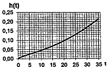
3-расм. Чўкма баландлигининг вақт (соат) бўйича ўзгариши.
