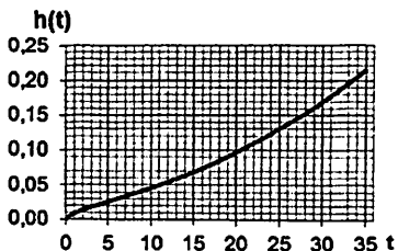
Рис. 3. Изменение слоя осадка по времени (час).
