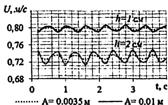
Рис. 1. Изменение скорости частиц в зависимости от времени.
