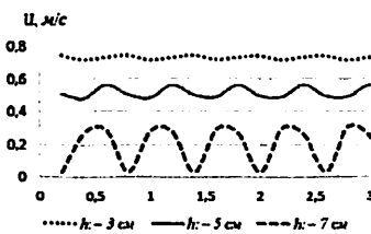
Рис. 2. Скорость частиц в зависимости от времени в различных слоях потока.
