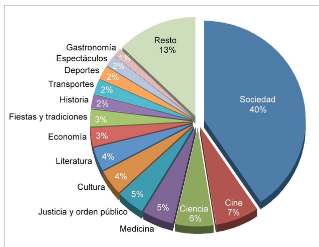
Gráfico 2. Distribución temática
