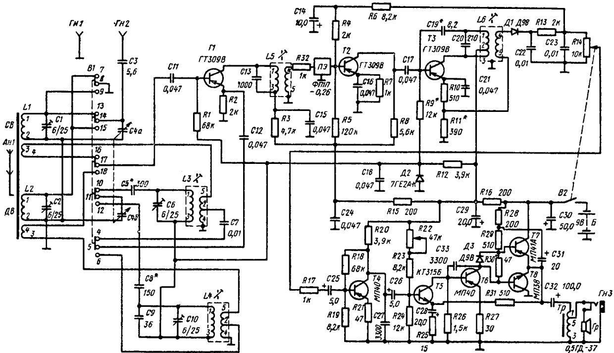
Принципиальная электрическая схема радиоприемника «Сокол-404»
